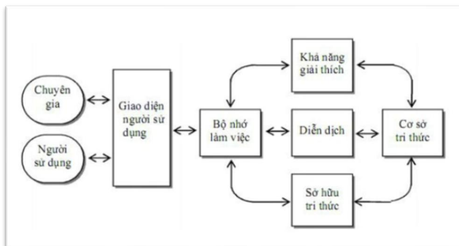
Hình 1.8 Kiến trúc hệ chuyên gia theo E.V.Popov
